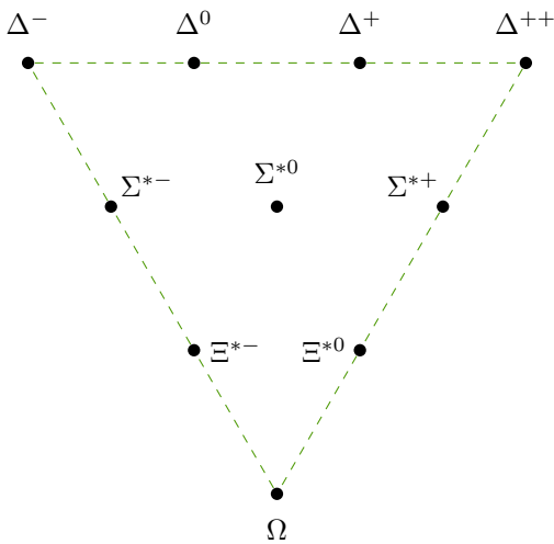
The Baryon Decuplet
