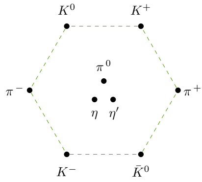
Pseudoscalar Meson Nonet (Octet plus Singlet \eta' )
