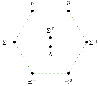
The Baryon Octet
